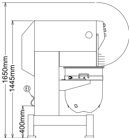
Oldalnézet
