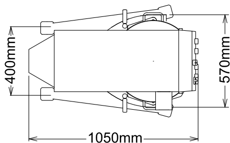
Felülnézet
